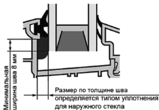
Рисунок 2 - Пример конструкции узла клею стеклопакета
