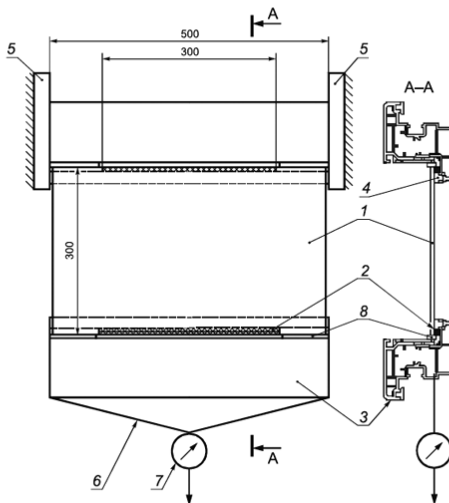
1 - наружное стекло; 2 - клеевой шов; 3 - профиль створки; 4 - уплотнительная прокладка; 5 - устройство крепления; 6 - устройство приложения нагрузки; 7 - динамометр; 8 - подкладка под стекло Рисунок 3 - Схема определения прочности клеевого соединения наружного стекла стеклопакета с наплавом створки
