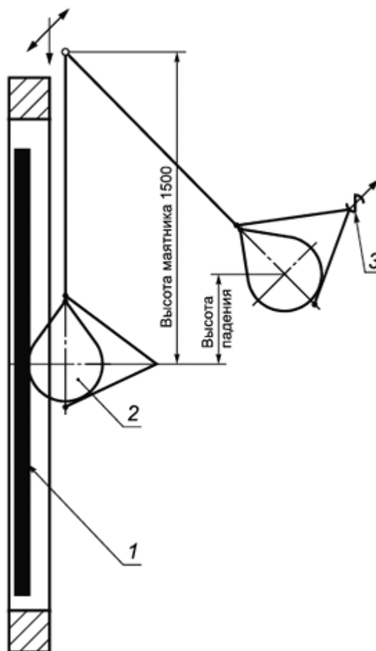
1 - испытуемый образец; 2 - груша (мягкое неупругое тело); 3 - съемный крюк Рисунок Ж.1 - Пример устройства для создания динамических нагрузок
