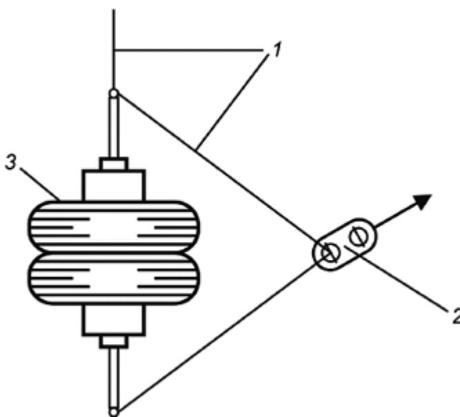
1 - трос; 2 - съемный крюк; 3 - груз Рисунок Ж.2 - Груз с двойными шинами массой (50,0 \pm 0,1) кг
